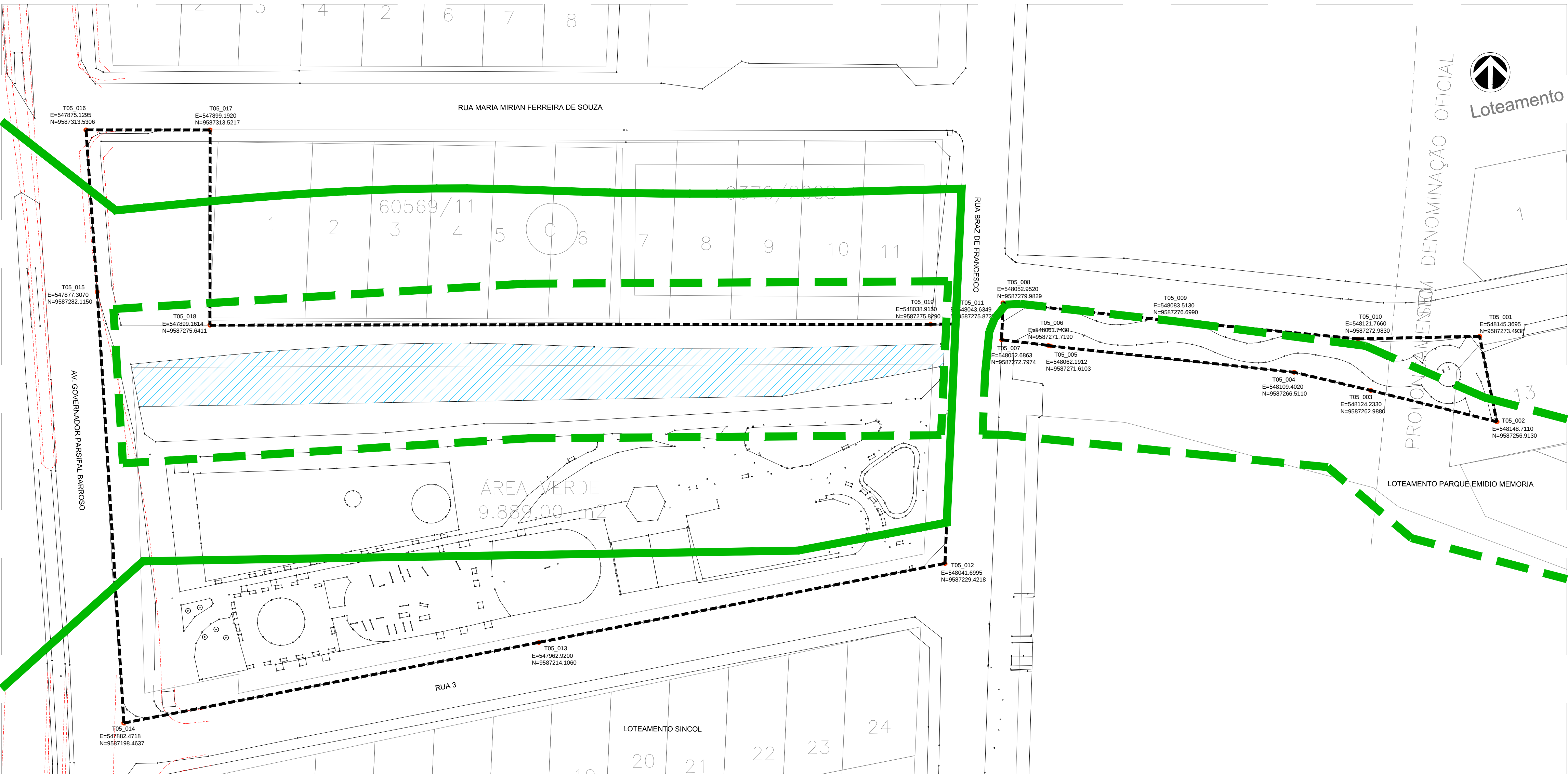
02 PLANTA DELIMITAÇÃO TRECHO 05 ESCALA 1/500
