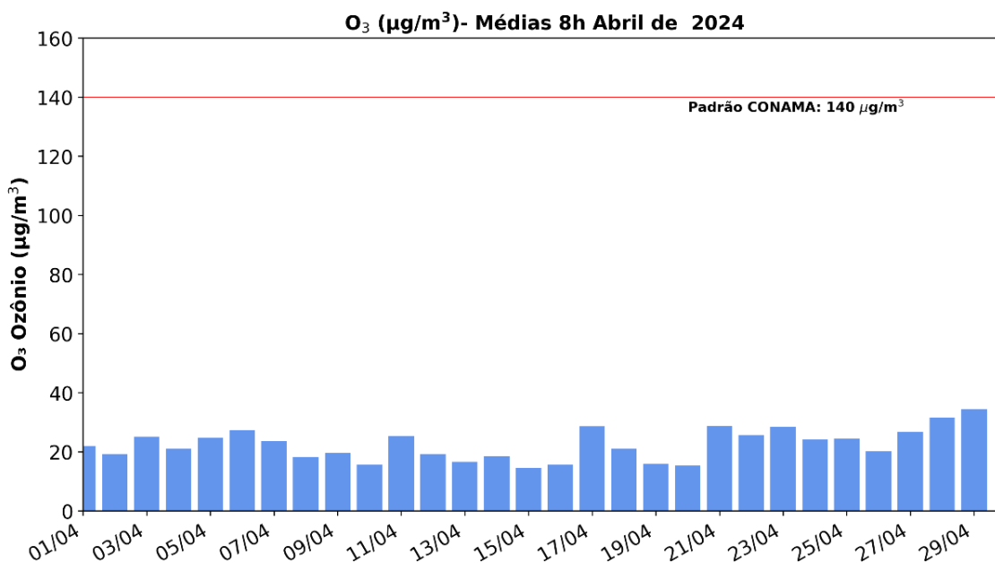
Figura 20: Concentrações médias móveis de 8h de O 3 na EMQAr em Abril de 2024.
