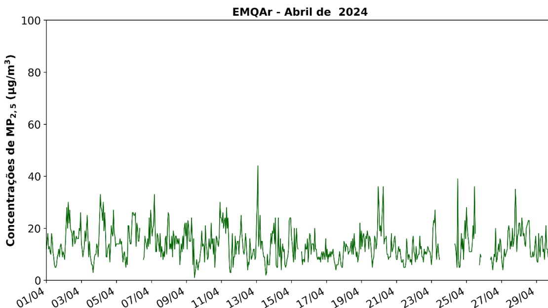
Figura 14: Concentrações médias horárias de \text{MP}_{2,5} na EMQAr em Abril de 2024.
