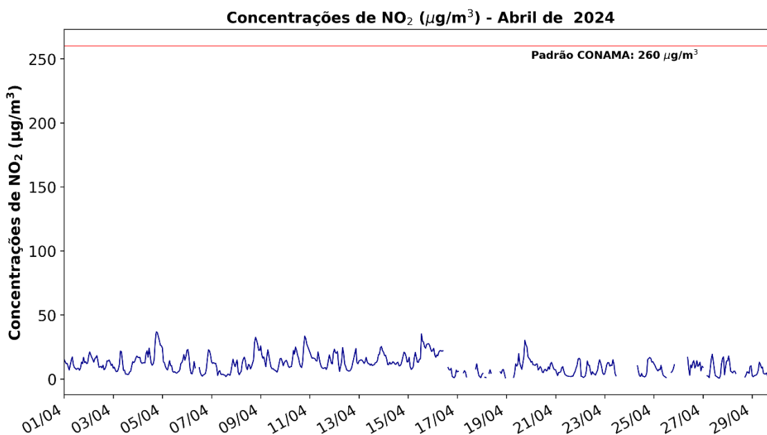
Figura 18: Concentrações médias horárias de NO 2 na EMQAr em Abril de 2024.
