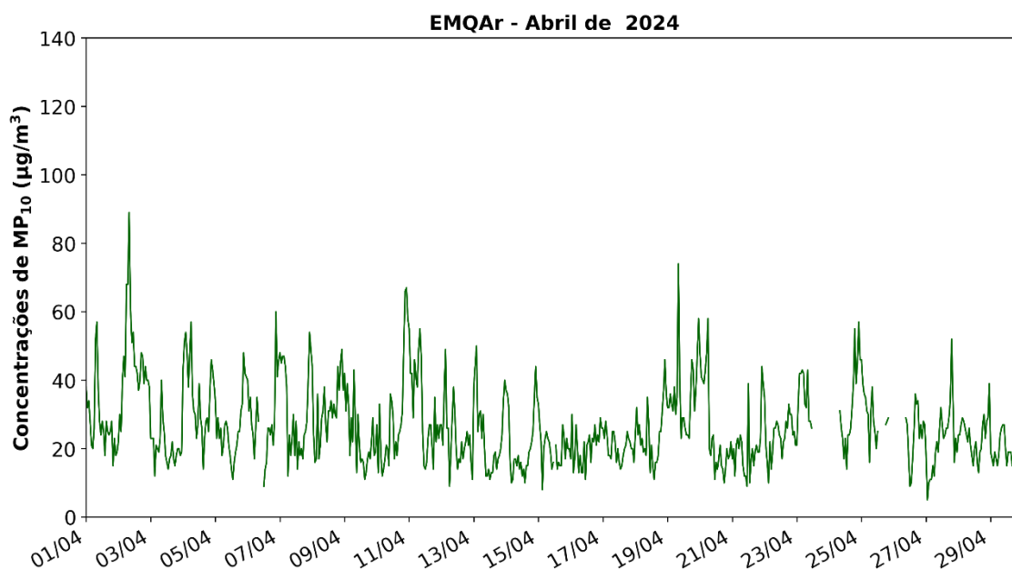
Figura 12: Concentrações médias horárias de MP 10 na EMQAr em Abril de 2024.
