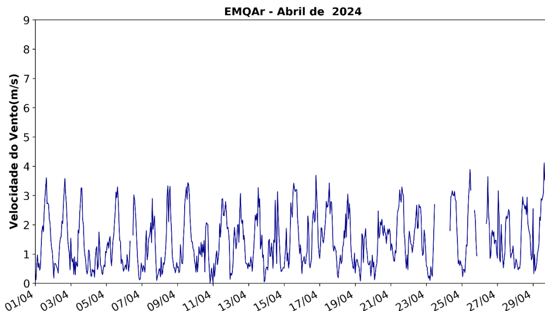
Figura 9: Registro da Velocidade do Vento na EMQAr em Abril de 2024.
