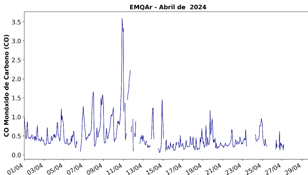
Figura 21: Concentrações médias horárias de CO na EMQAr em Abril de 2024.
