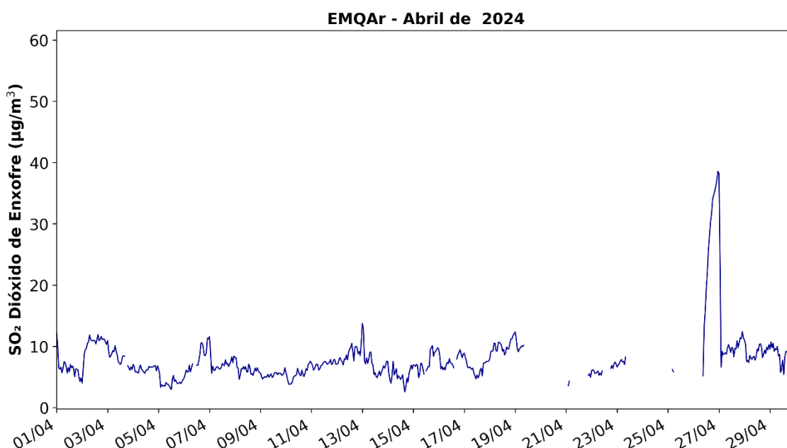
Figura 16: Concentrações médias horárias de SO 2 na EMQAr em Abril de 2024.
