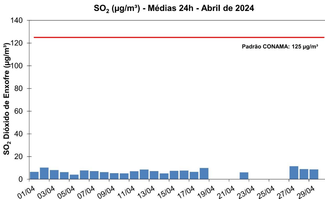
Figura 17: Concentrações médias diárias de SO 2 na EMQAr em Abril de 2024.
