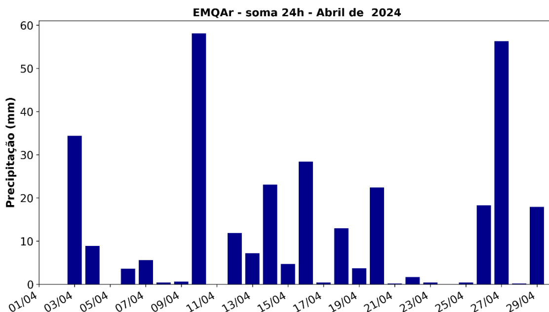
Figura 5: Precipitação acumulada diária na EMQAr em Abril de 2024.
