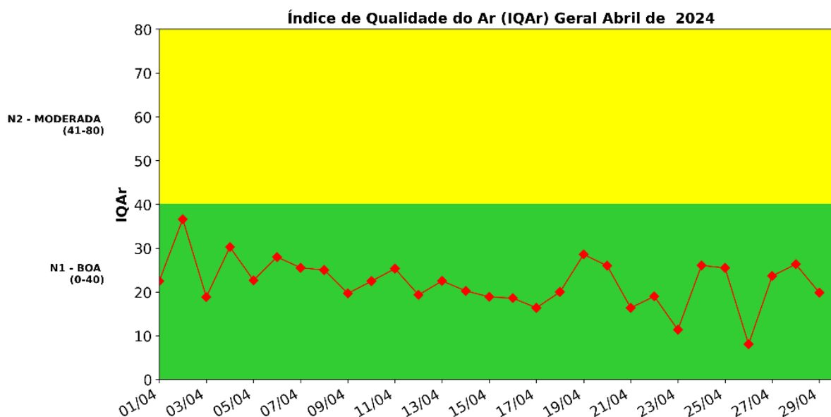
Figura 23: Índice de qualidade do ar na EMQAr em Abril de 2024.
