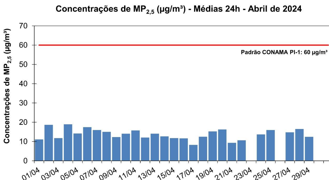
Figura 15: Concentrações médias diárias MP 2,5 na EMQAr em Abril de 2024.
