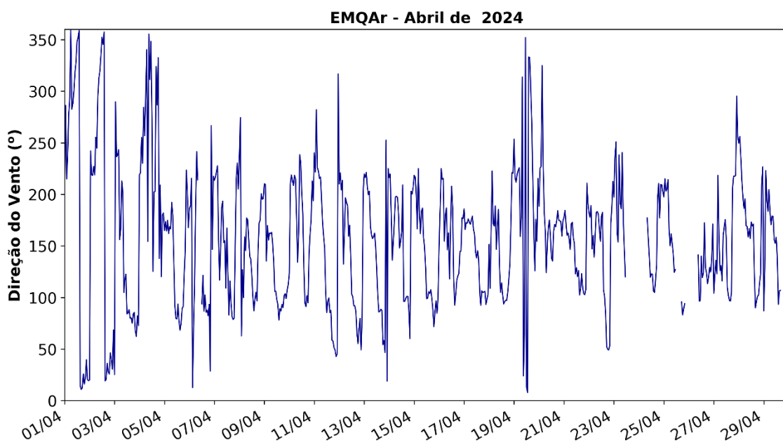
Figura 10: Registro da Direção do Vento na EMQAr em Abril de 2024.
