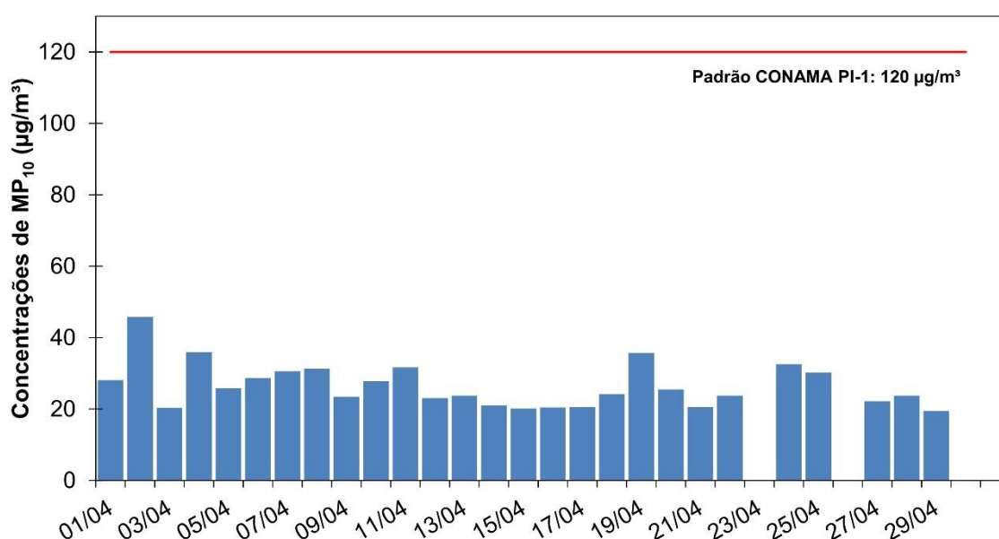
Figura 13: Concentrações médias diárias de MP 10 na EMQAr em Abril de 2024.
