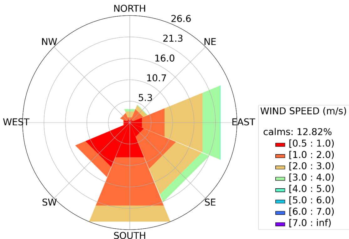
Figura 11: Rosa dos Ventos na EMQAr em Abril de 2024.
