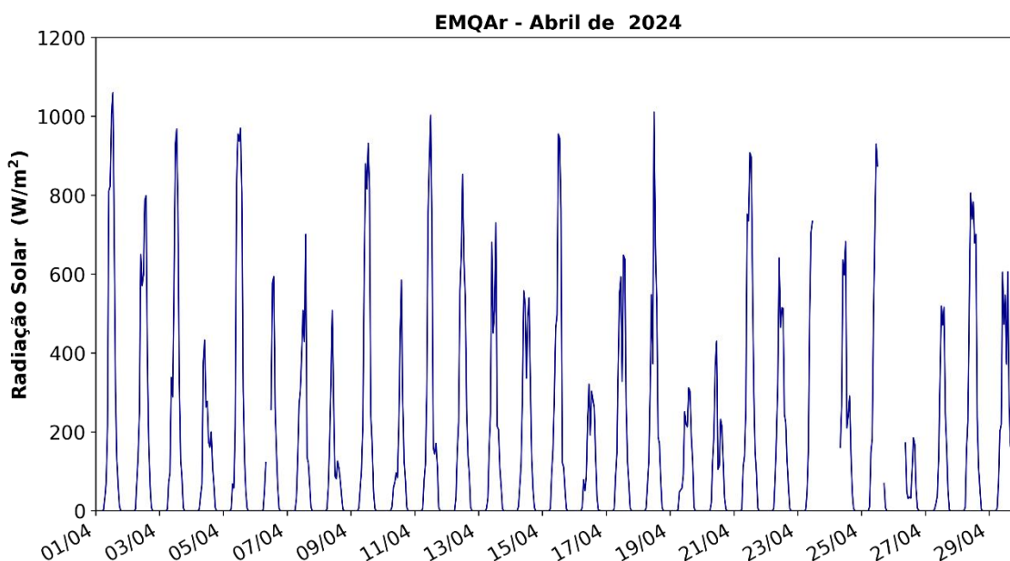
Figura 8: Registro da Radiação Solar na EMQAr em Abril de 2024.
