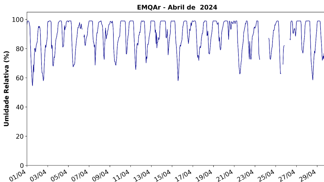
Figura 6: Registro da Umidade Relativa do Ar na EMQAr em Abril de 2024.
