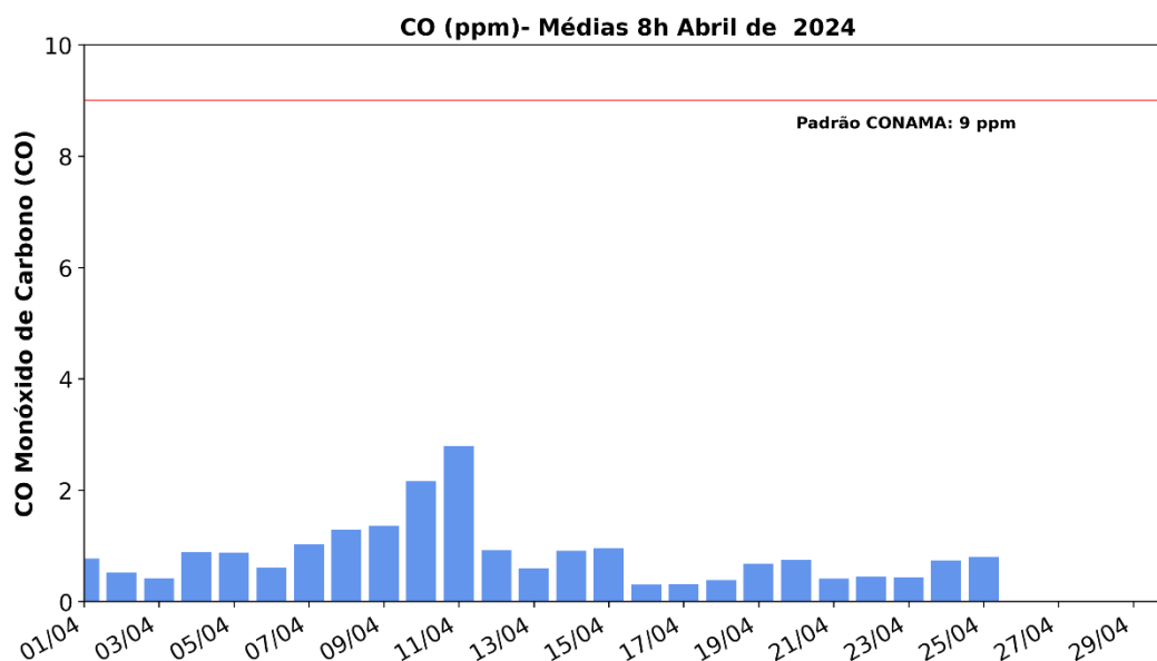
Figura 22. Concentrações médias móveis de 8h de CO na EMQAr em Abril de 2024.
