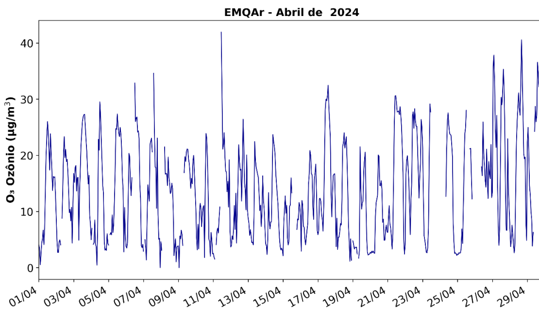
Figura 19: Concentrações médias horárias de \text{O}_3 na EMQAr em Abril de 2024.
