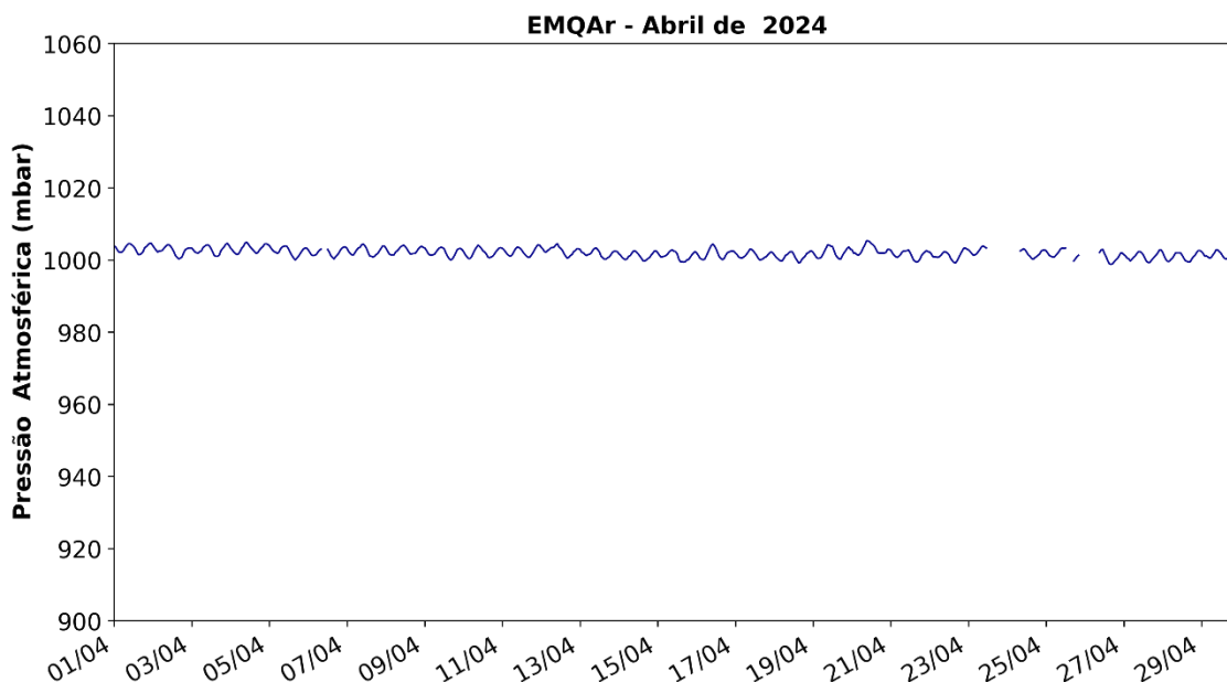
Figura 7: Registro da Pressão Atmosférica na EMQAr em Abril de 2024.
