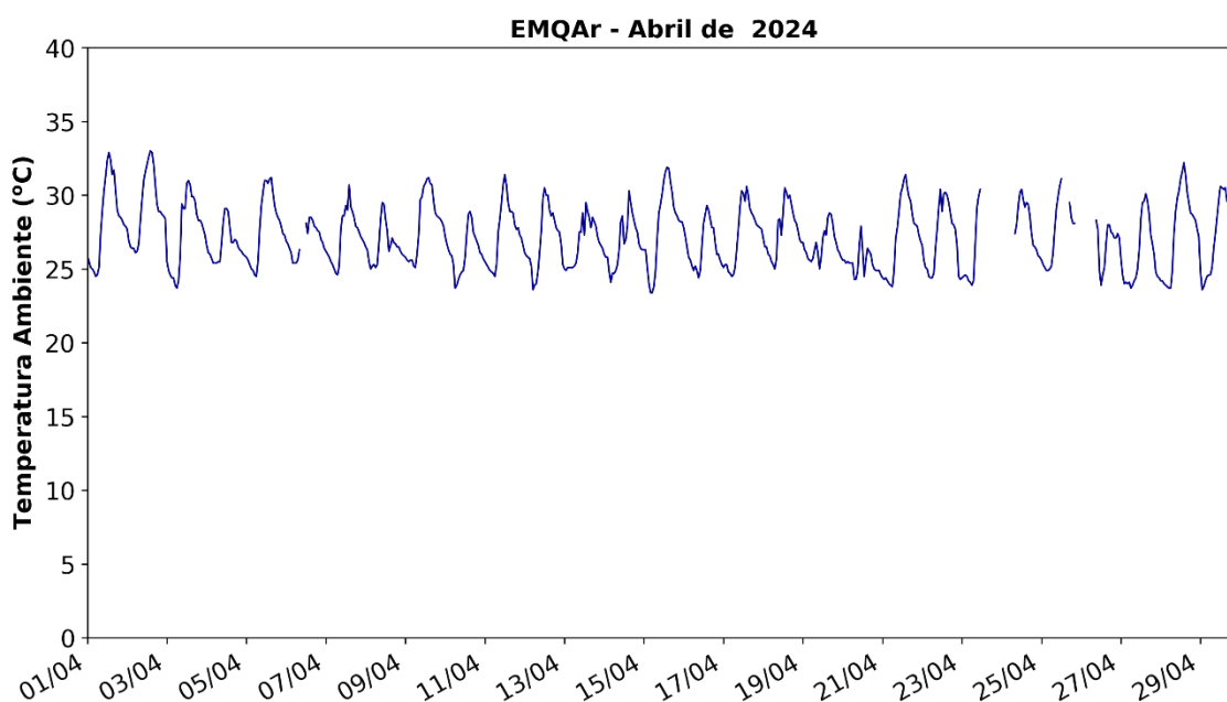
Figura 3: Registro da Temperatura Ambiente na EMQAr em Abril de 2024.
