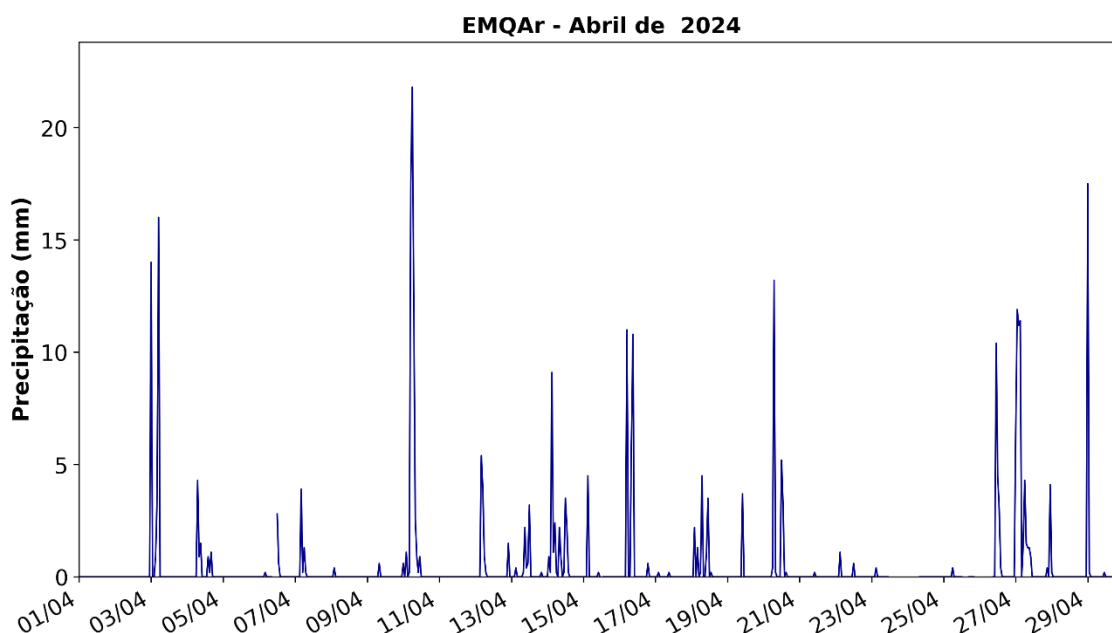
Figura 4: Registro da Precipitação Pluviométrica na EMQAr em Abril de 2024.
