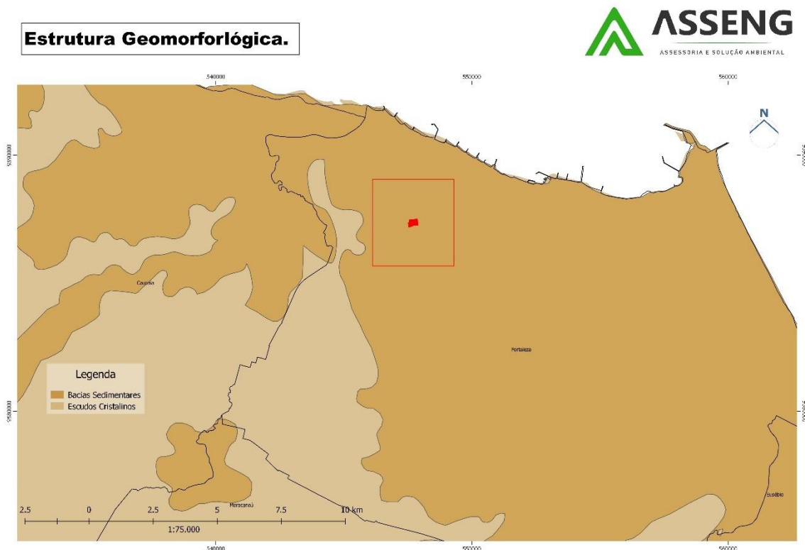
Figura 4.2 - Estrutura geológica, trecho 6.
