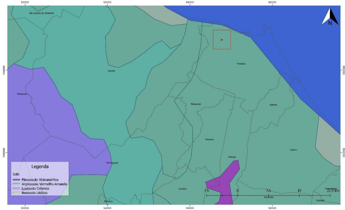
Figura 4.3 - Tipos de solo, trecho 6. Fonte: Adaptado de IBGE - EMBRAPA, 2001.
