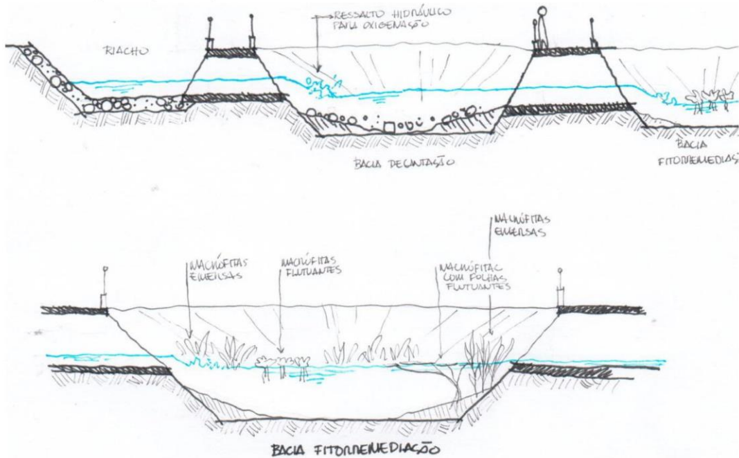
Cortes esquemáticos de funcionamento do sistema de wetlands. Fonte: produzido pelos autores, 2016.
